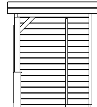
(R) Zijaanzicht / Side view / Seiten ansicht
